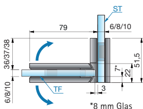
Glasudskæring til 8 mm glas uden tætningsliste
