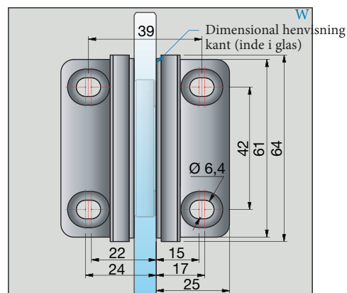
Monteringsplade 8134ZN
