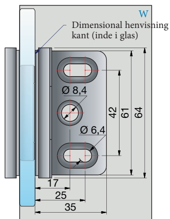
Monteringsplade 8130ZN
