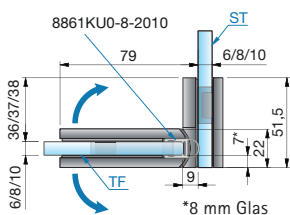
Glasudskæring til 8 mm glas med tætningsliste 8861KU0-8-2010
