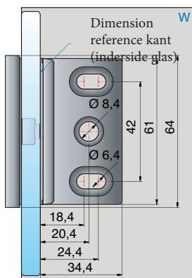
Monteringsplade 8194ZN
