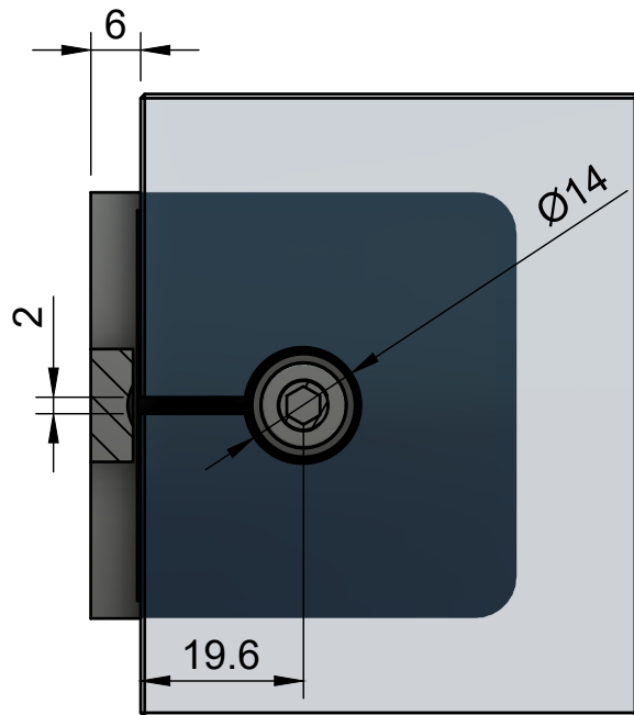
Glas med Ø14 hul og teknisk Cut
