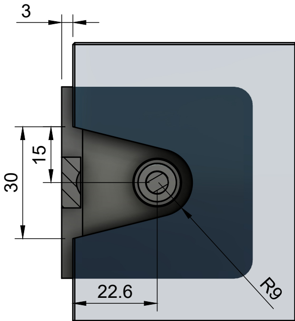
Glas med Udfræsning
